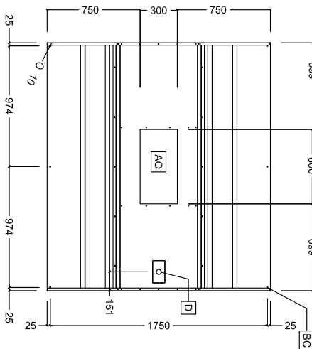
Boven aanzicht
